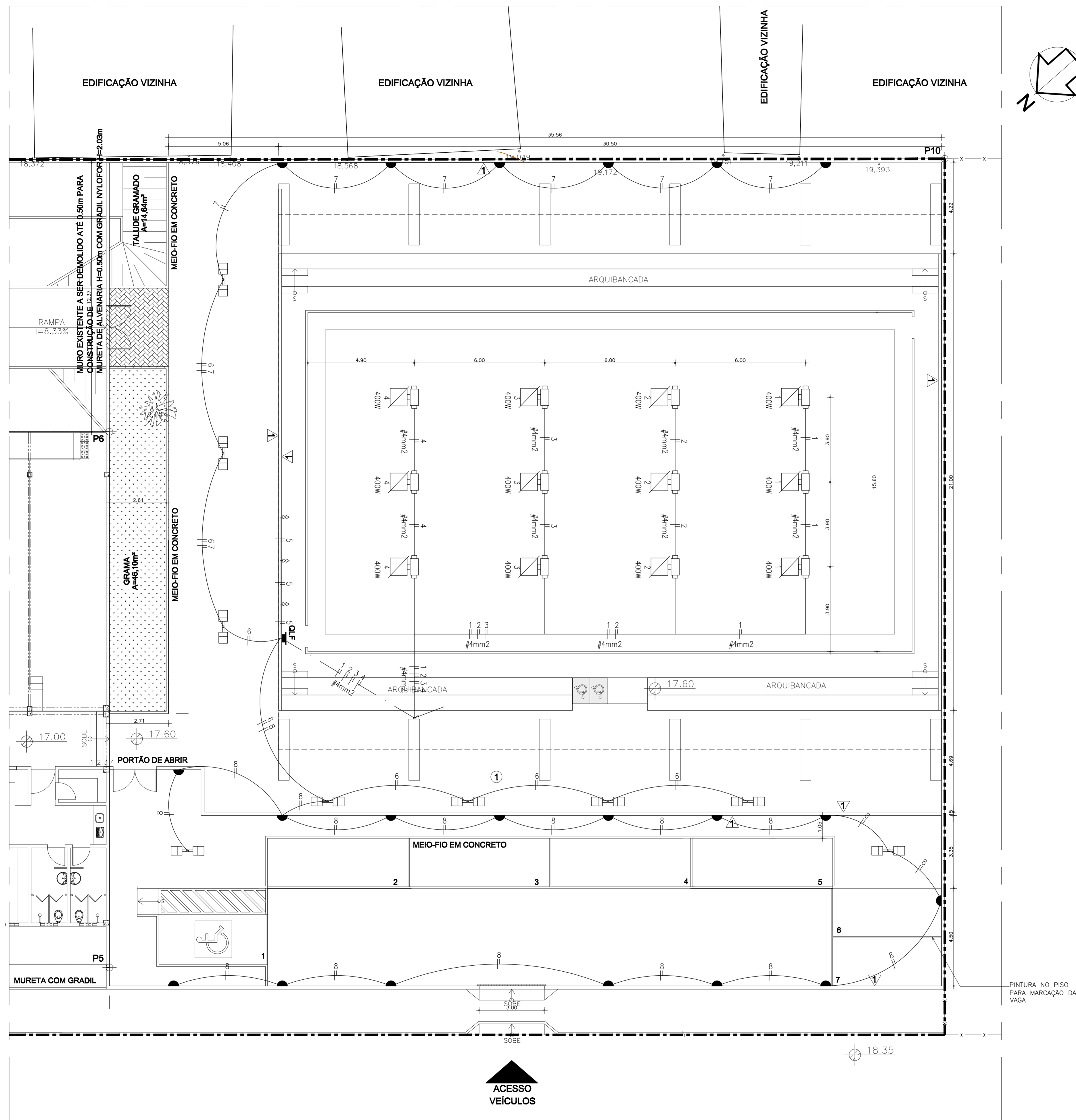
1 PROJ. ELÉTRICO QUADRA E ESTACIONAMENTO ESC.: 1:100
